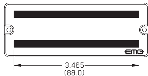
EMG-40CS/40DC
